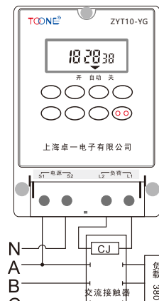
图 3 三相负载
