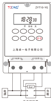
图 2 单相负载
