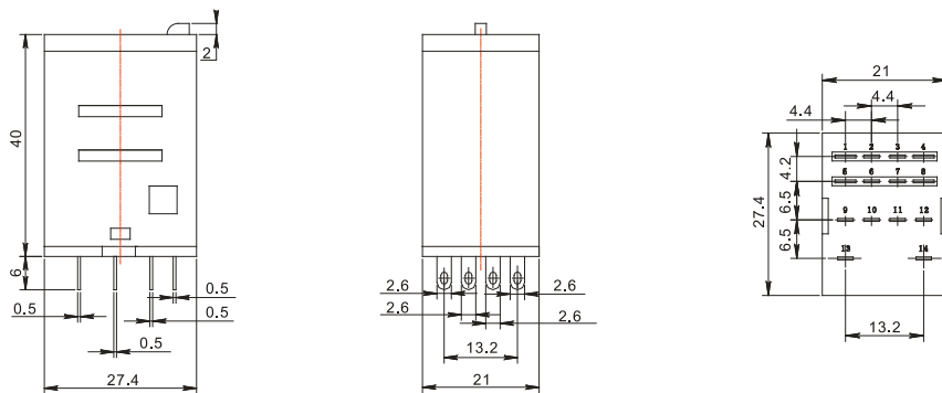
ZYR3-MY4LT 插拔式
