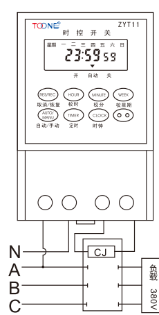
交流接触器 三相负载 图 3
