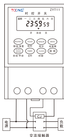
单相负载 图 2
