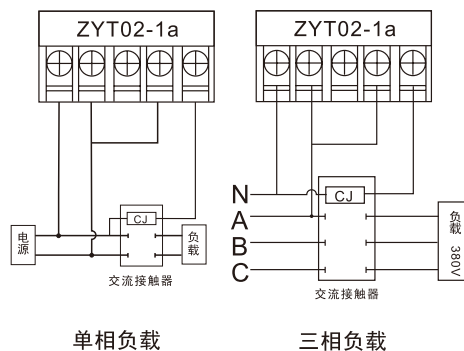
单相负载
