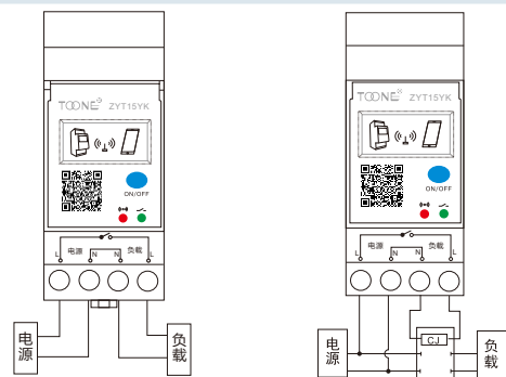
图1 直接接线
