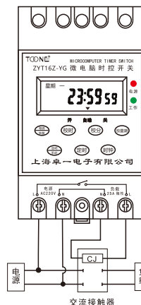
图 2 单相负载
