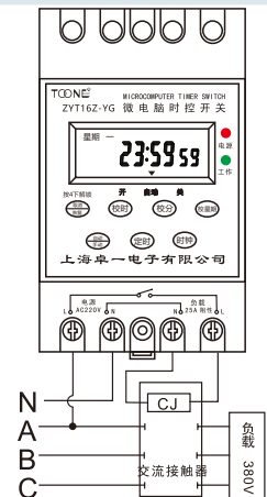
图 3 三相负载
